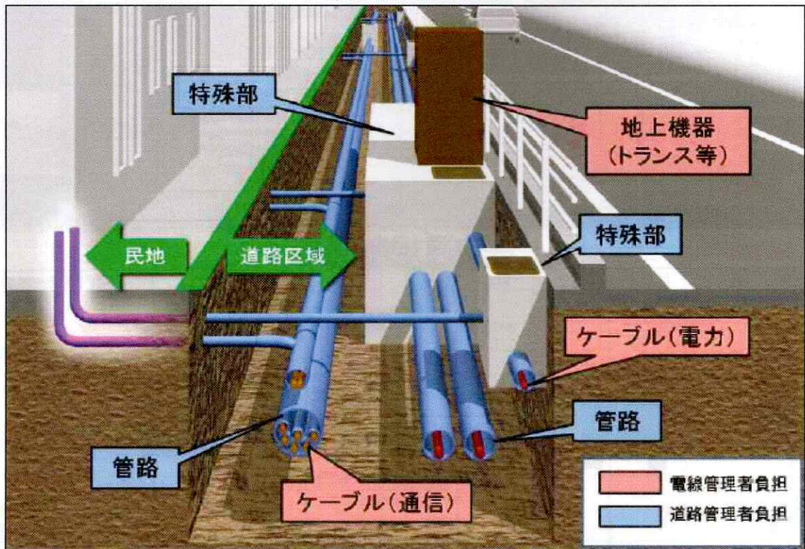
< 電線共同溝イメージ >
